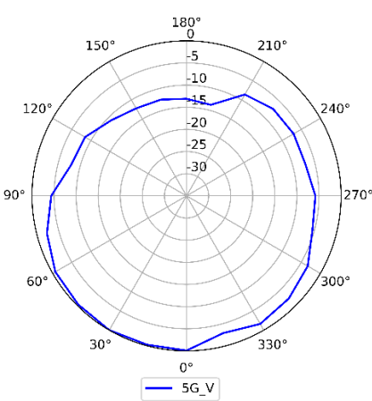
5GHz (Vertical)
