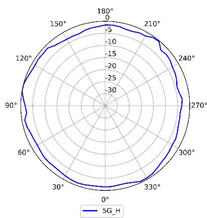
5GHz (Horizontal)
